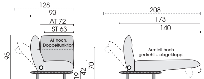
Seitenansicht M240DFH
